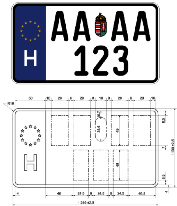
2. ábra: „B” típusú rendszámtábla rajzai
