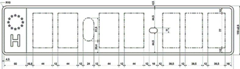
1. ábra: „A” és „D” típusú rendszámtáblák rajzai
