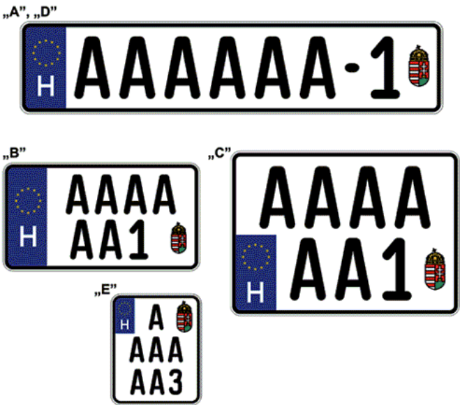
9. ábra: A tagállamjelzés, a címer és a karakterek elrendezése az egyedileg előállított rendszámtáblákon
