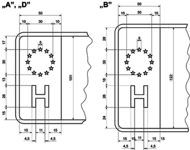
6. ábra: „A”, „D” és „B” típusú rendszámtáblák tagállamjelzésének méretei
