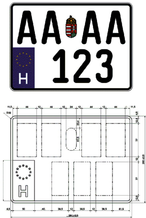
3. ábra: „C” típusú rendszámtábla rajzai
