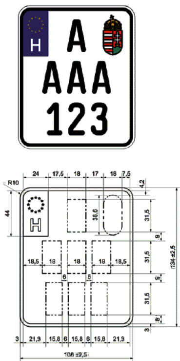
4. ábra: „E” típusú rendszámtábla rajzai
