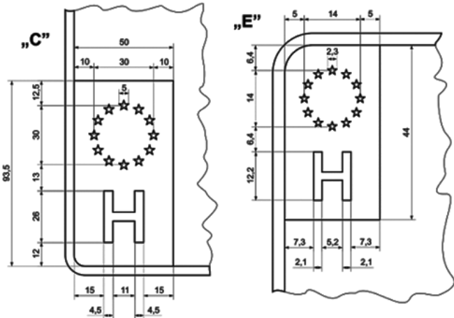
7. ábra: „C” és „E” típusú rendszámtáblák tagállamjelzésének méretei
